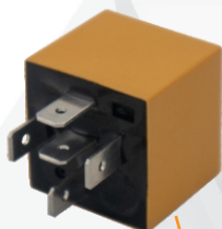
رله تهویه هوای زرد ۳۵ آمپر (پژو/سمند/پارس)
